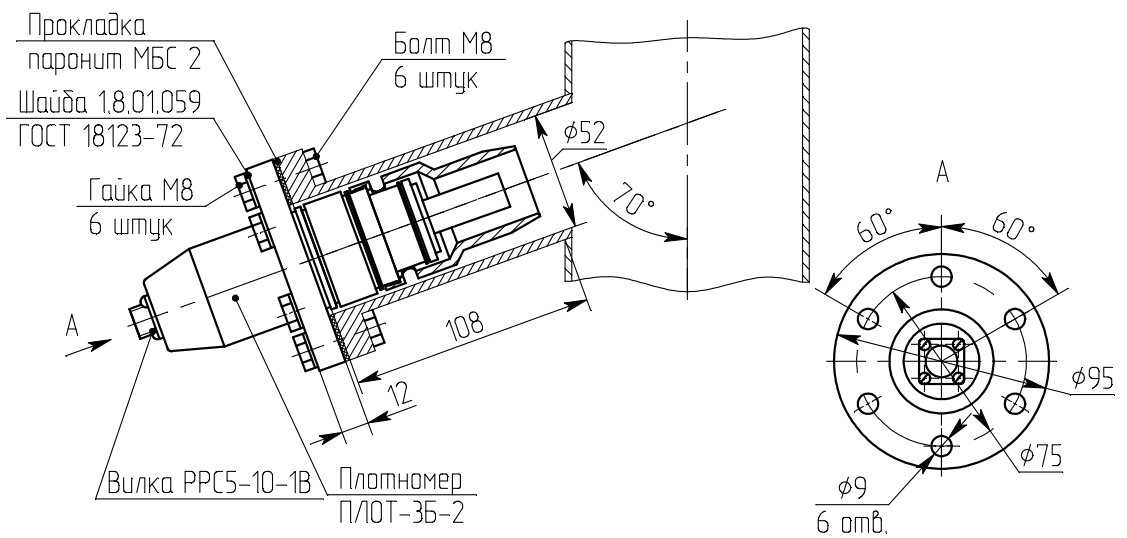
б) на вертикальном трубопроводе
